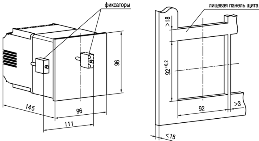
Рисунок Б.1 – Габаритные и установочные размеры ТРМ32-Щ4
