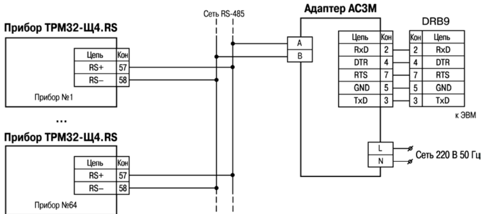
Рисунок В.3 – Схема подключения TPM32-Щ4.01.RS и TPM32-Щ4.03.RS к адаптеру сети AC3M
