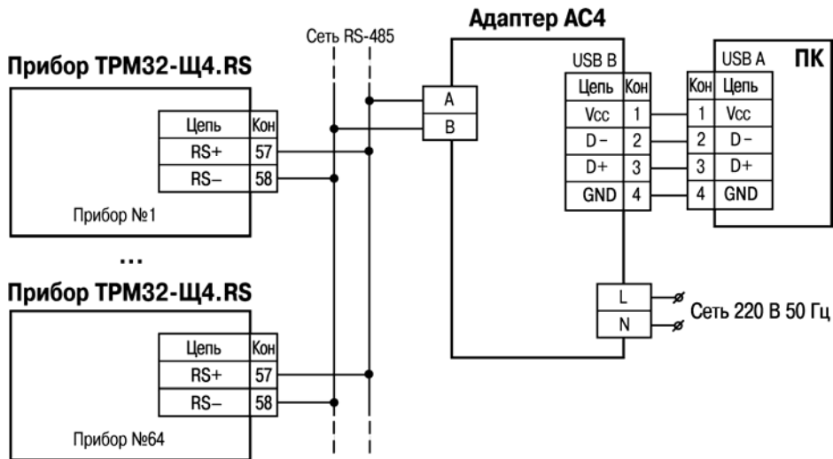
Рисунок В.3 – Схема подключения TPM32-Щ4.01.RS и TPM32-Щ4.03.RS к адаптеру сети АС4
